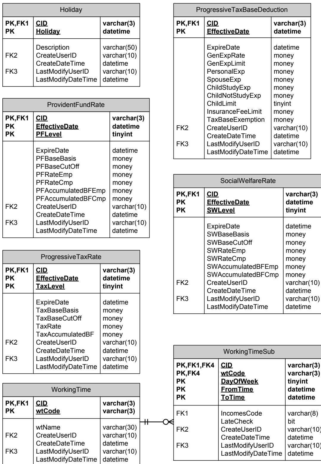
รูปที่ 2.9 แผนภาพ ER-Diagram ของกลุ่มข้อมูลค่าติดตั้งของการคำนวณค่าจ้าง (บางส่วน)
