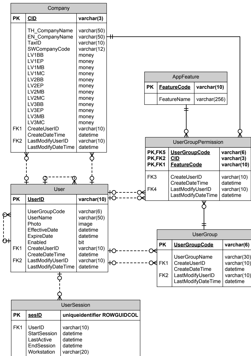
รูปที่ 2.2 แผนภาพ ER-Diagram ของกลุ่มข้อมูลผู้ใช้
