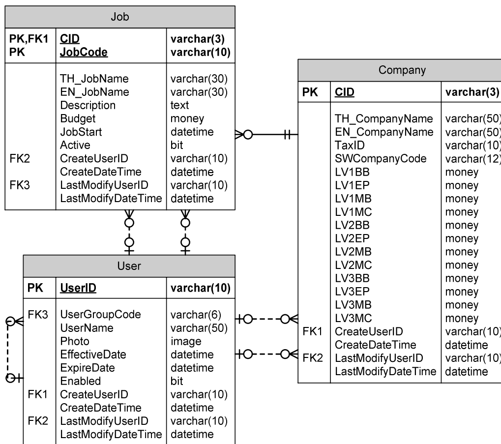
รูปที่ 2.8 แผนภาพ ER-Diagram ของกลุ่มข้อมูลงาน
