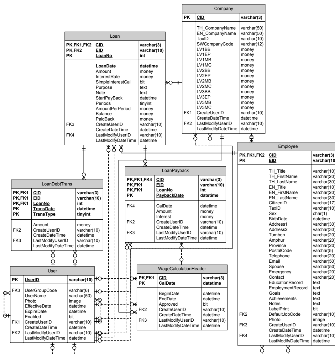
รูปที่ 2.11 แผนภาพ ER-Diagram ของกลุ่มข้อมูลการกู้ยืมเงิน
