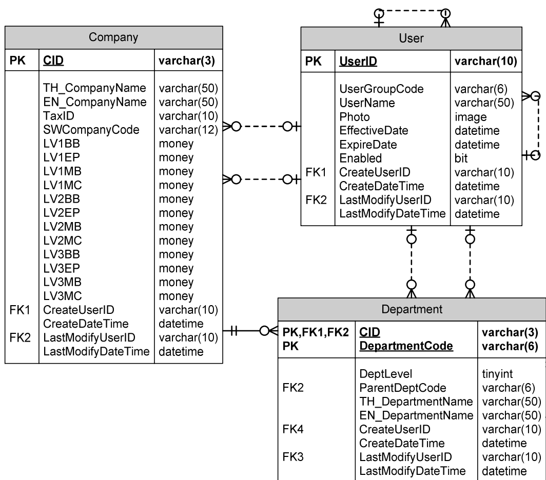
รูปที่ 2.4 แผนภาพ ER-Diagram ของกลุ่มข้อมูลฝ่าย
