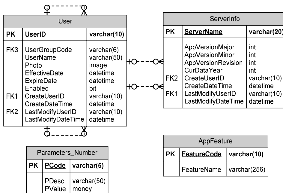
รูปที่ 2.3 แผนภาพ ER-Diagram ของกลุ่มข้อมูลโปรแกรม
