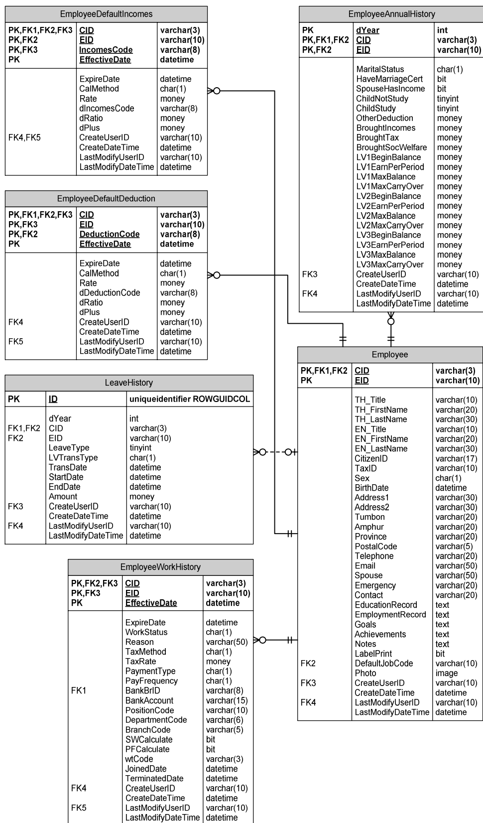
รูปที่ 2.7 แผนภาพ ER-Diagram ของกลุ่มข้อมูลพนักงาน
