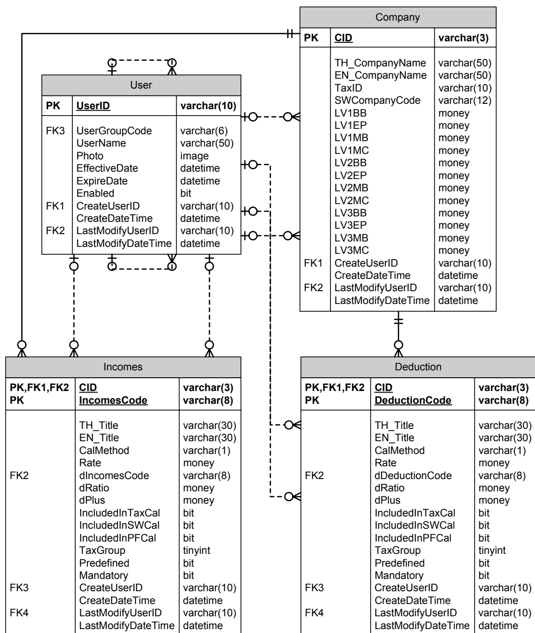
รูปที่ 2.10 แผนภาพ ER-Diagram ของตารางรายได้และรายจ่าย
