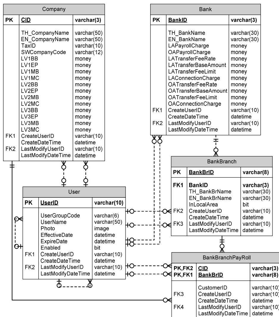
รูปที่ 2.6 แผนภาพ ER-Diagram ของกลุ่มข้อมูลธนาคาร
