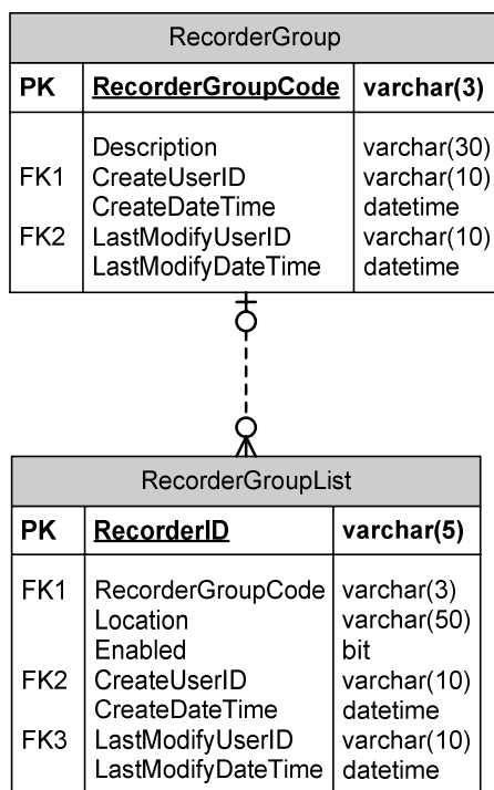
รูปที่ 2.15 แผนภาพ ER-Diagram ของกลุ่มข้อมูลเครื่องบันทึกเวลา
