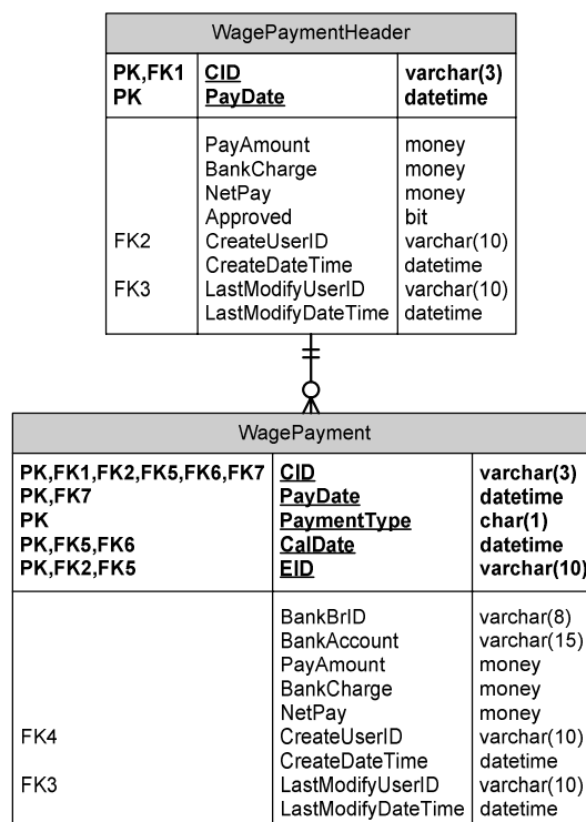
รูปที่ 2.13 แผนภาพ ER-Diagram ของกลุ่มข้อมูลการจ่ายค่าจ้าง
